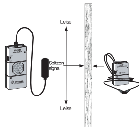
Abb. 07 - Nachweis von Bohrstellen
