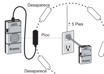
Fig. 03 - Rastreo en las Paredes
