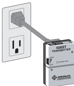
Figure 1 - Fiche d'adaptateur secteur
