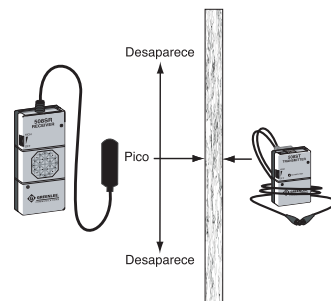
Fig. 07 – Localización Exacta de Sitios de Perforación
