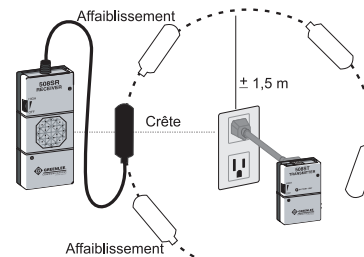
Figure 3 - Suivi du cheminement derrière des murs
