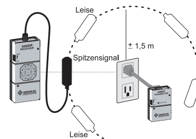
Abb. 03 - Verfolgung von Unterputzleitungen
