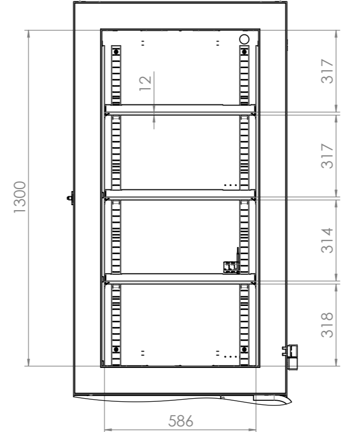
Y 1 : 15 Ansicht ohne Tür view without door
