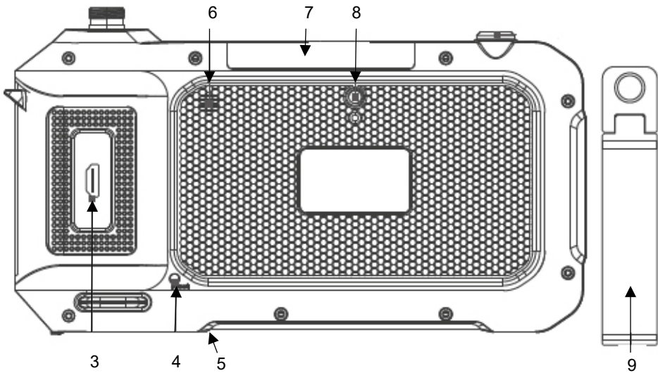
Abb. 3: Geräte-Rückseite
