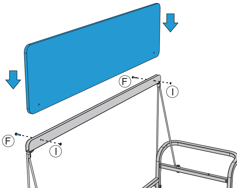
Sign Coroplast 1x
