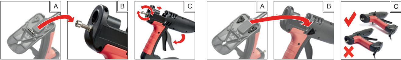
El perno suministrado se puede utilizar para ajustar el recorrido del gatillo.
