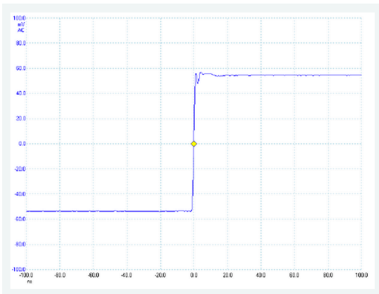
Abbildung 3: Gute Kompensation
