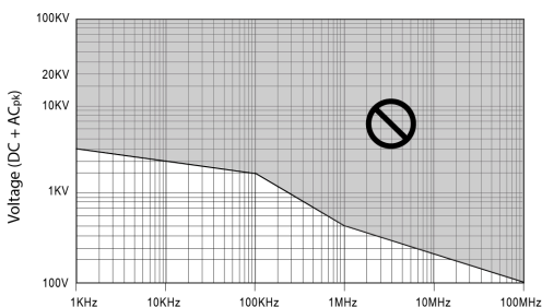
Figure 4: Courbe de limitation de la tension en fonction de la fréquence
