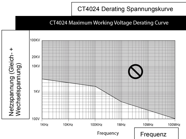
Abbildung 4: Derating Spannungskurve
