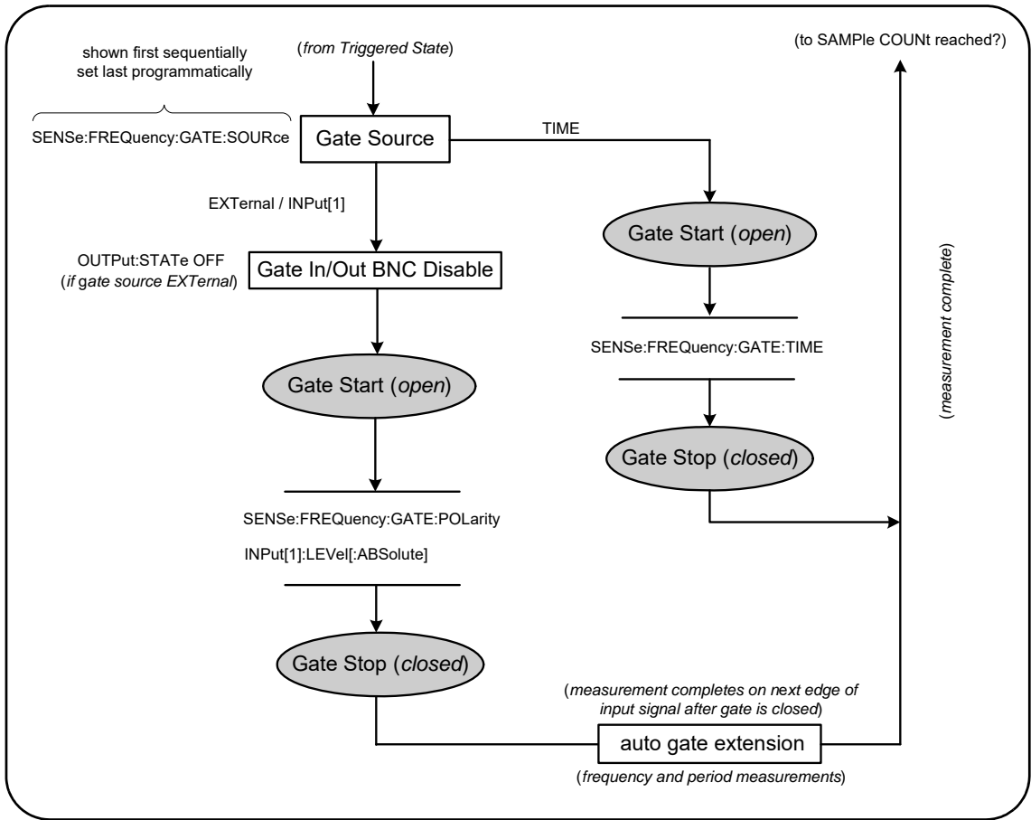
Figure 5-2 (suite) Cycle de déclenchement et de porte - Commutation de porte
