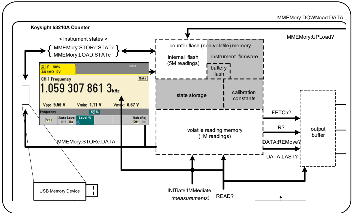
Figure 7-1 Flux de données dans le compteur 53210A
