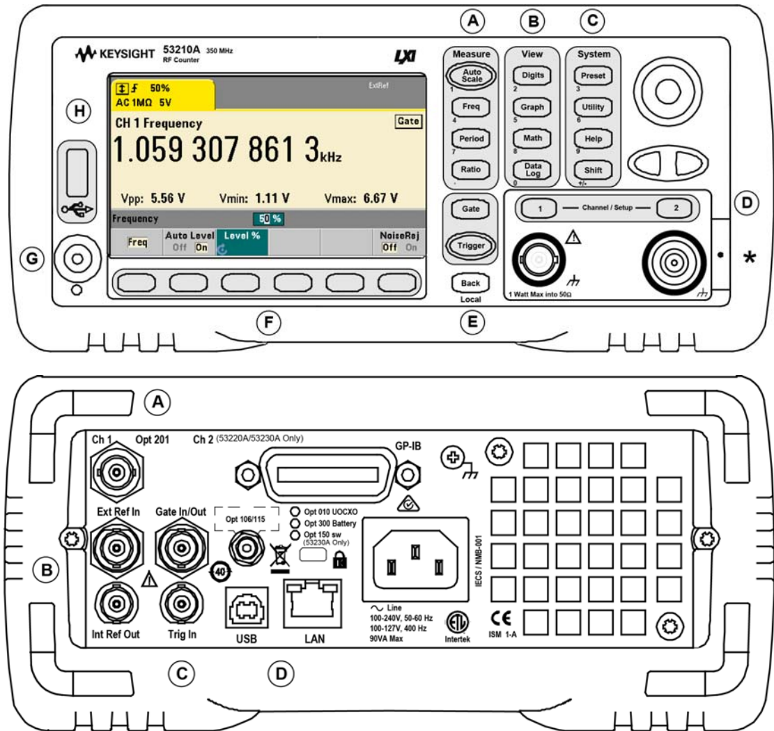
Figure 1-1 Compteur/fréquenceur universel 53210A.
