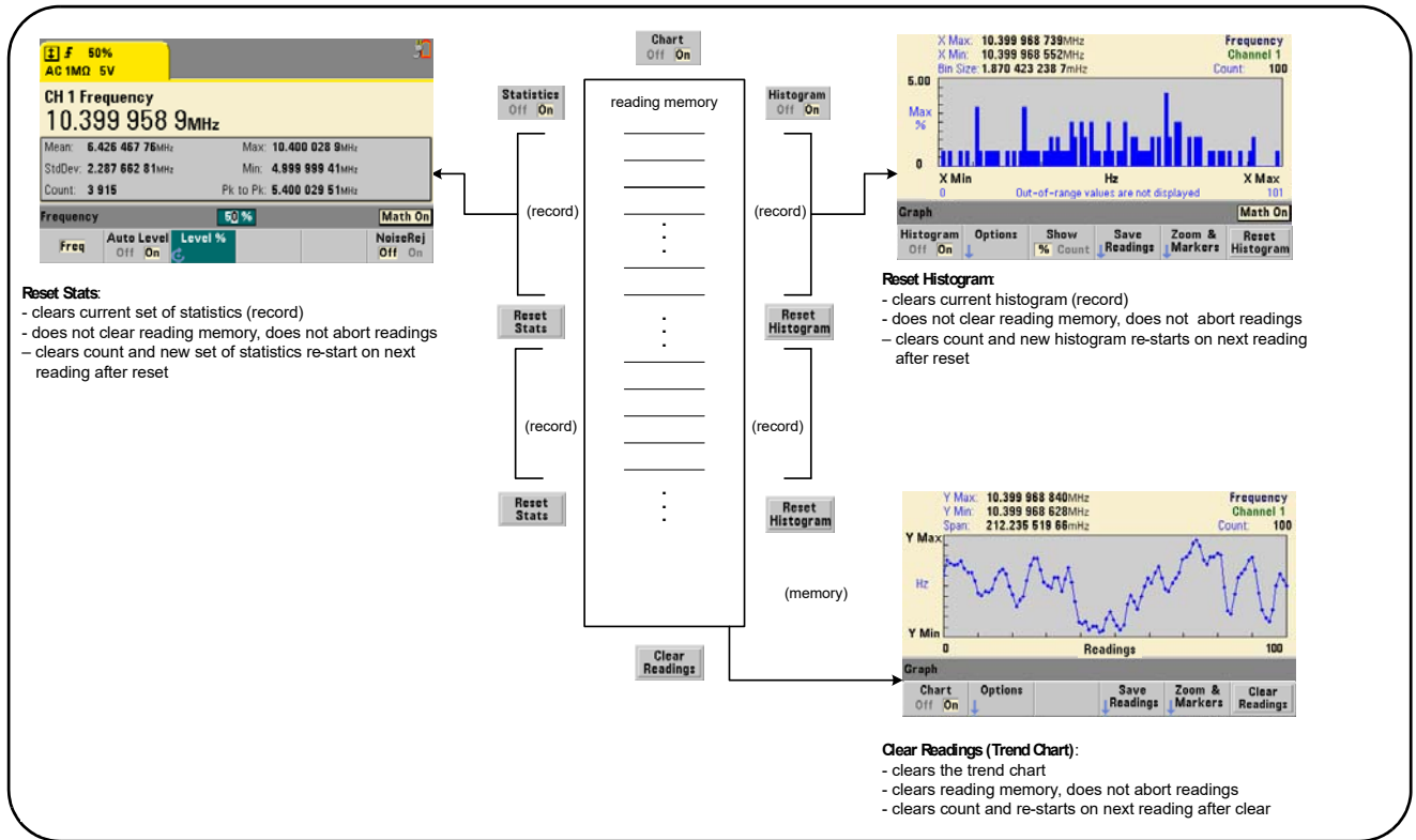
Figure 6-13 Mémoire de mesures et remise à zéro/effacement des graphes
