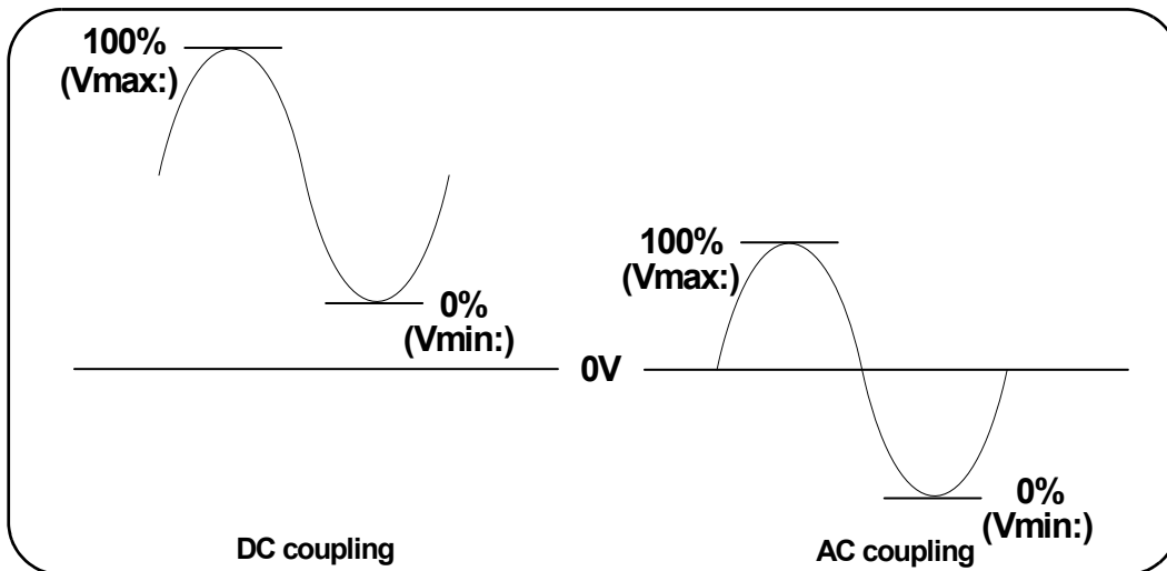
Figure 4-5 Couplage d'entrée et niveaux de seuil et relatifs
