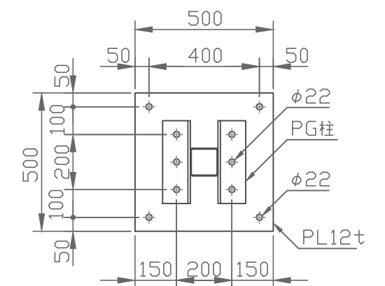
ベースプレート詳細
