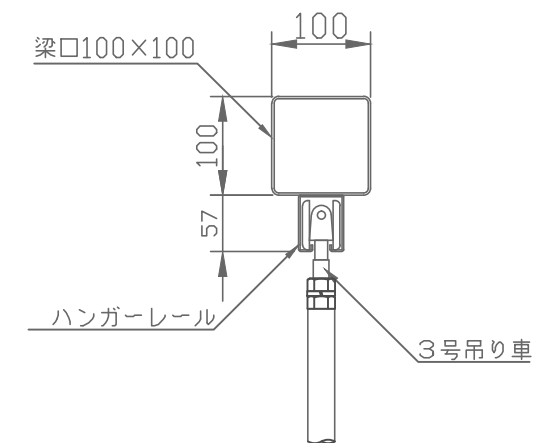
吊り車部詳細
