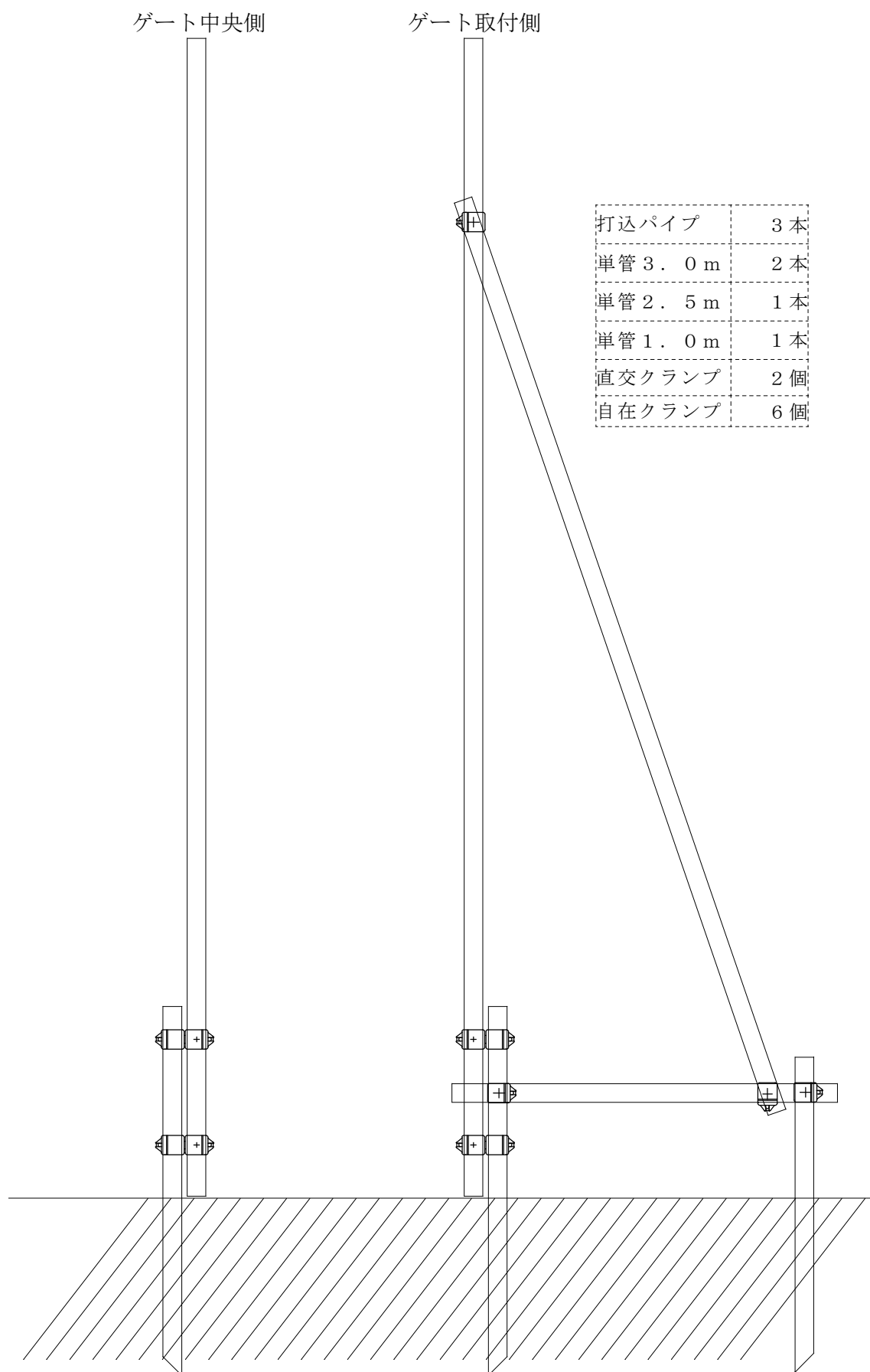
【 P C G N 取付用 単管組立図 】
