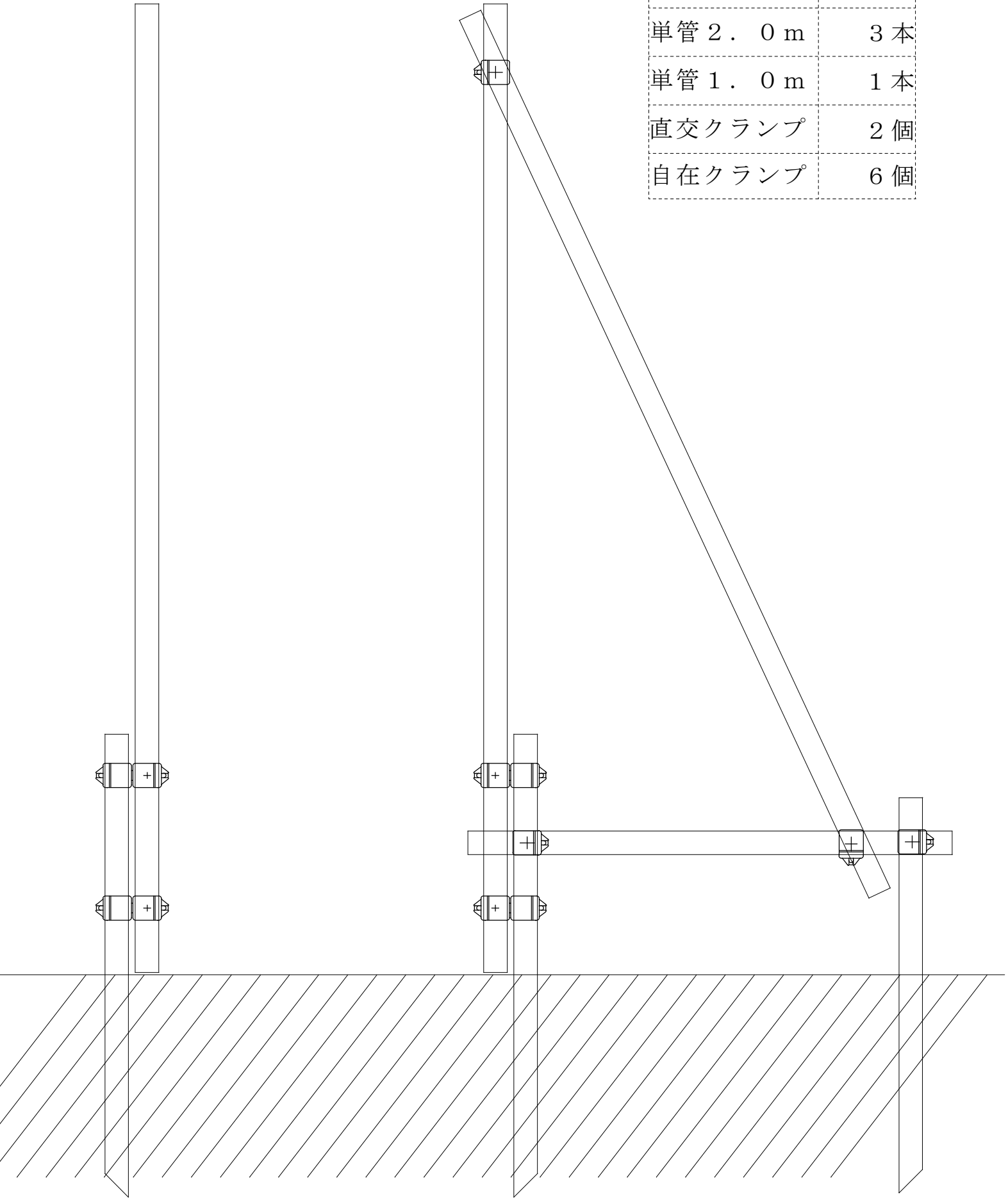
【 P C G ・ H C G 取付用 単管組立図 】
