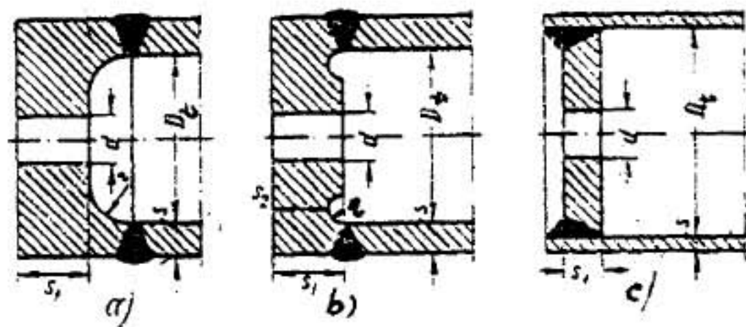
Hình 2 - Cách nối đáy phẳng với thân hình trụ
