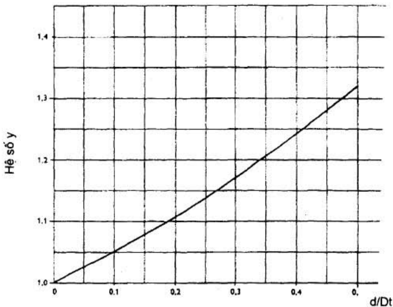
Hình 8 - Xác định hệ số hiệu chỉnh y
