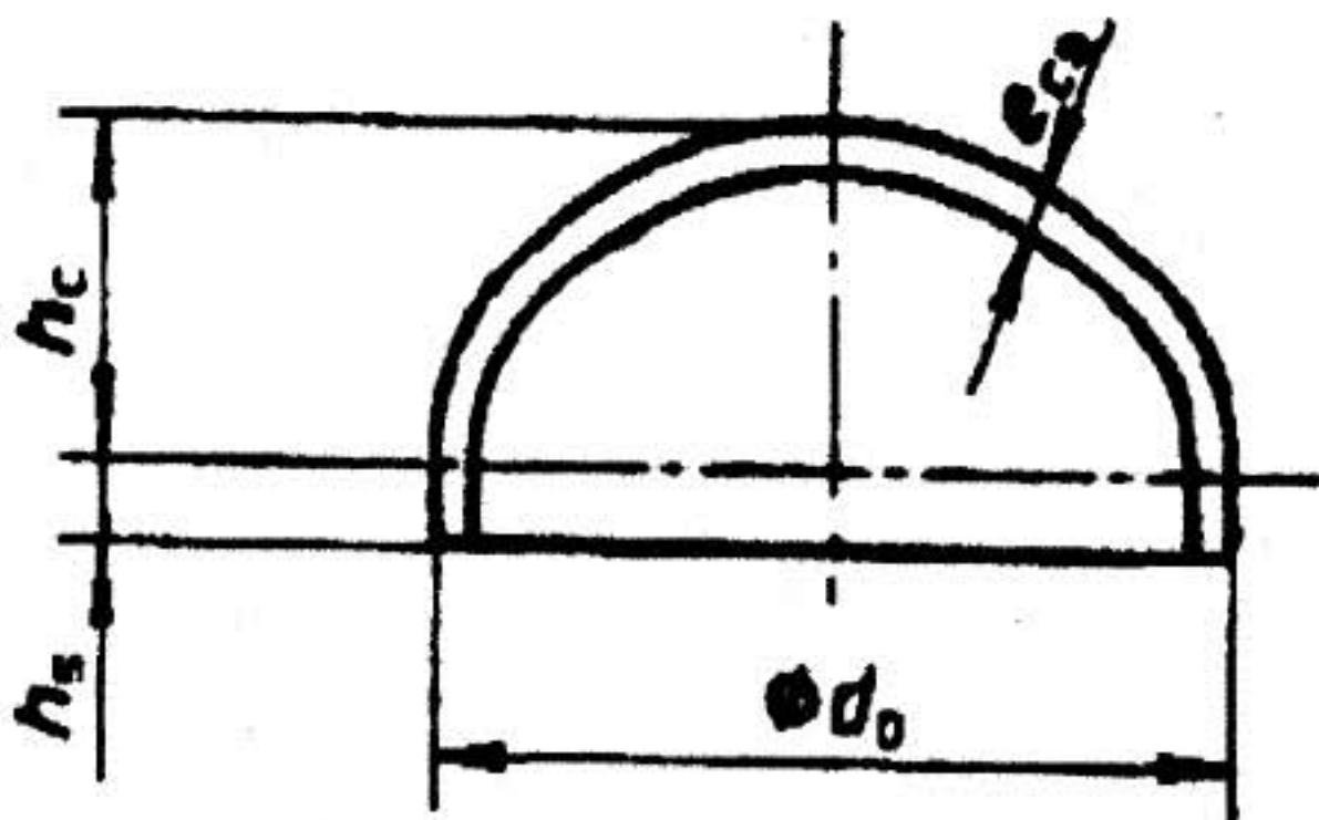
Hình 3 - Cấu tạo đáy elíp
