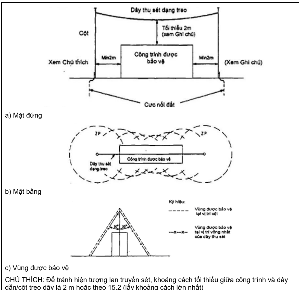
Hình 17 - Bộ phận thu sét và vùng bảo vệ công trình đơn giản có chứa chất dễ cháy nổ
