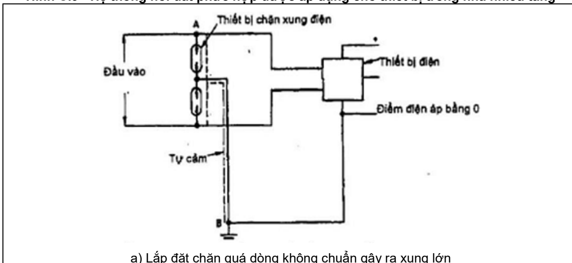
Hình C.9 - Hệ thống nối đất phức hợp được áp dụng cho thiết bị trong nhà nhiều tầng
