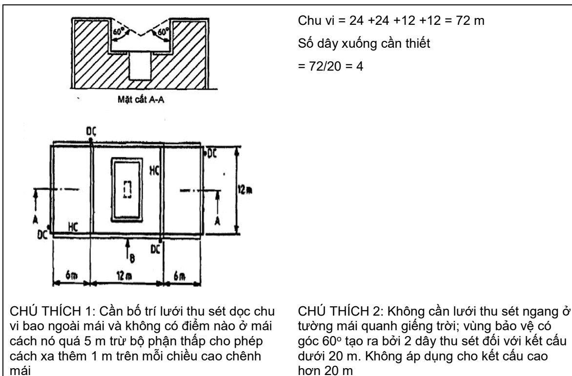
Hình 10 - Thu sét cho mái bằng có nhiều độ cao khác nhau
