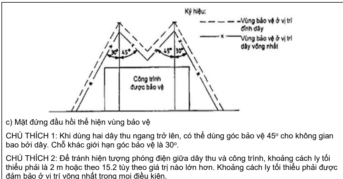
Hình 30 - Bộ phận thu sét có hai dây thu sét treo ngang và vùng bảo vệ cho kết cấu có chứa chất nổ hoặc chất rất dễ cháy
