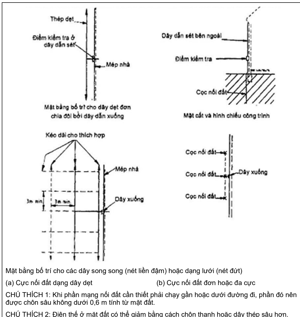
Hình 24 - Mạng nối đất: bố trí các cực nối đất
