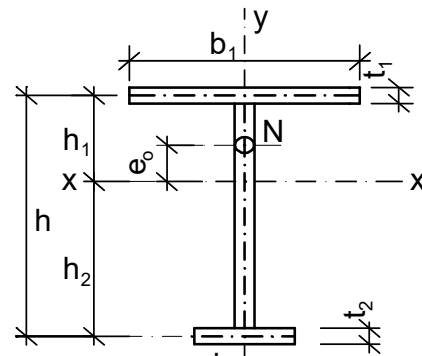
Hình D.4 – Sơ đồ tiết diện chữ I một trục đối xứng chịu nén lệch tâm
