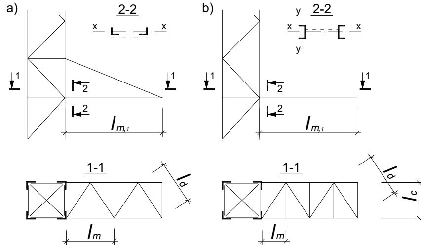
Hình 21 – Sơ đồ xà ngang
