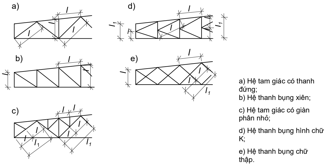
Hình 8 – Các sơ đồ thanh bụng giàn để xác định chiều dài tính toán các thanh
