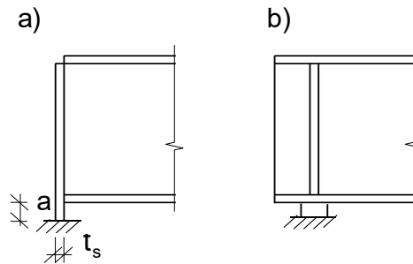
Hình 12 – Sơ đồ đặt sườn cứng ở gối
