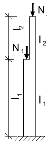
HÌNH D.1 □ SƠ ĐỒ CỘT MỘT
