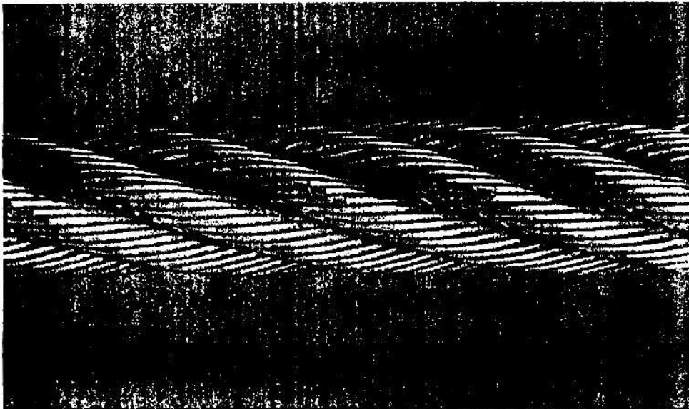
Hình B.13 – Đứt sợi vùng lồi
