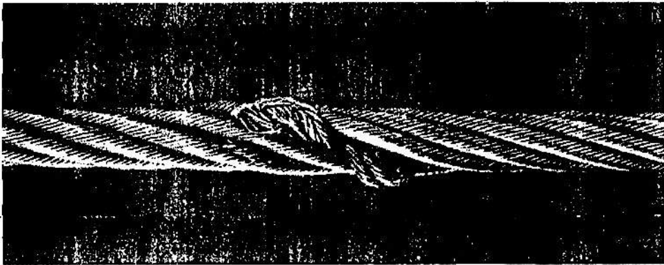
Hình B.2 – Lõi nhô ra – cáp cuộn một lớp
