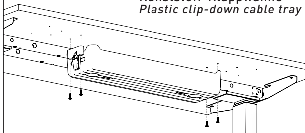
Klappwanne öffnen Open clip-down cable tray
