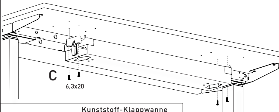
Kunststoff-Klappwanne Plastic clip-down cable tray
