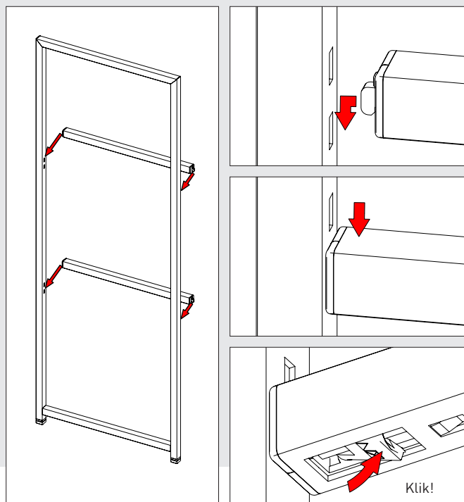
7 | KLIK-VERBINDINGSTECHNIEK voor verbinding van ladder en dwarsbuis.
