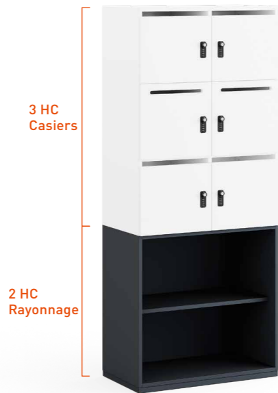
RAYONNAGE ACTA.PLUS AVEC ARMOIRES À CASIER À SUPERPOSER Rayonnage 2 HC et armoire à casiers 3 HC P : 600 mm, L : 800 mm Serrure à combinaison et fente pour courrier
