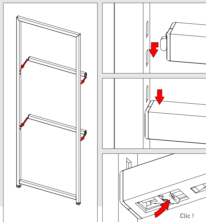
7 | TECHNIQUE DE LIAISON PAR ENCLIQUETAGE pour relier les échelles aux barreaux.
