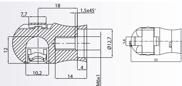
7266 RÓTULA - BALLCUP - ROTULE
