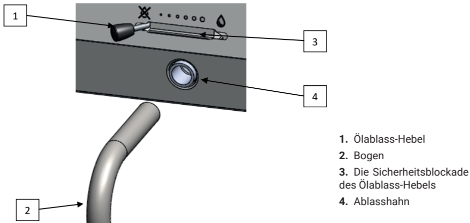
Bild 9 Die Elemente des Ölablassmechanismus
