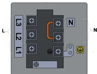
Bild 6. Anschluss des Gerätes an die elektrische Installation
