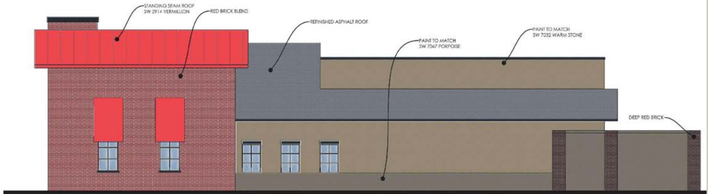
RIGHT ELEVATION
