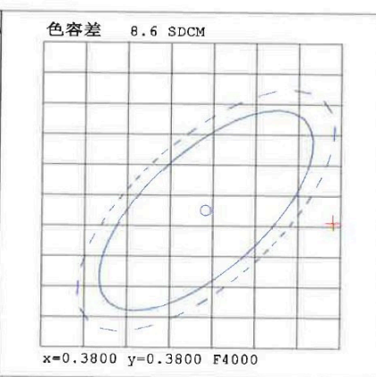
CIE1931色品图
