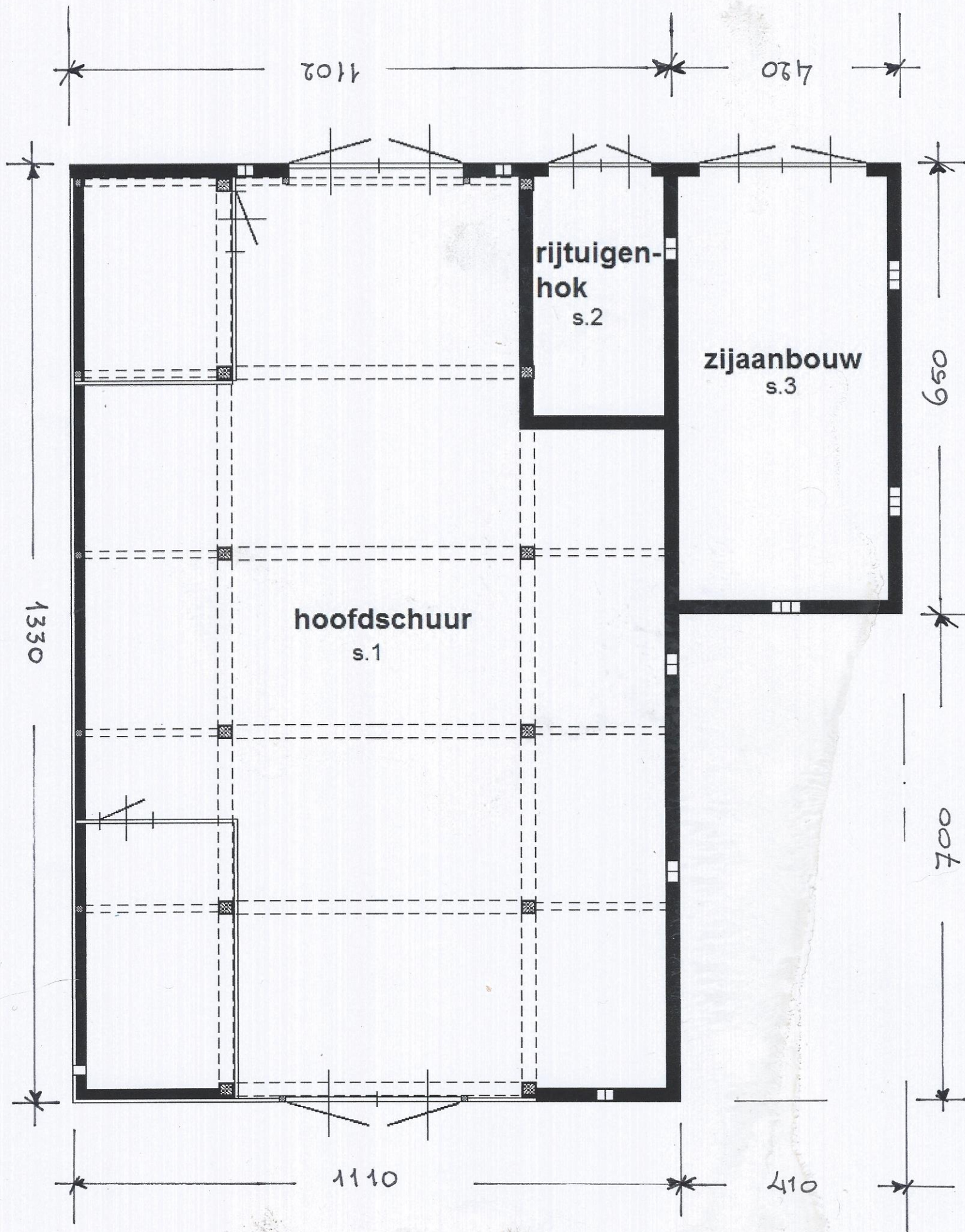
HOOFDMATEN SCHUUR KEUNENHUIS. MATEN IN CM.
