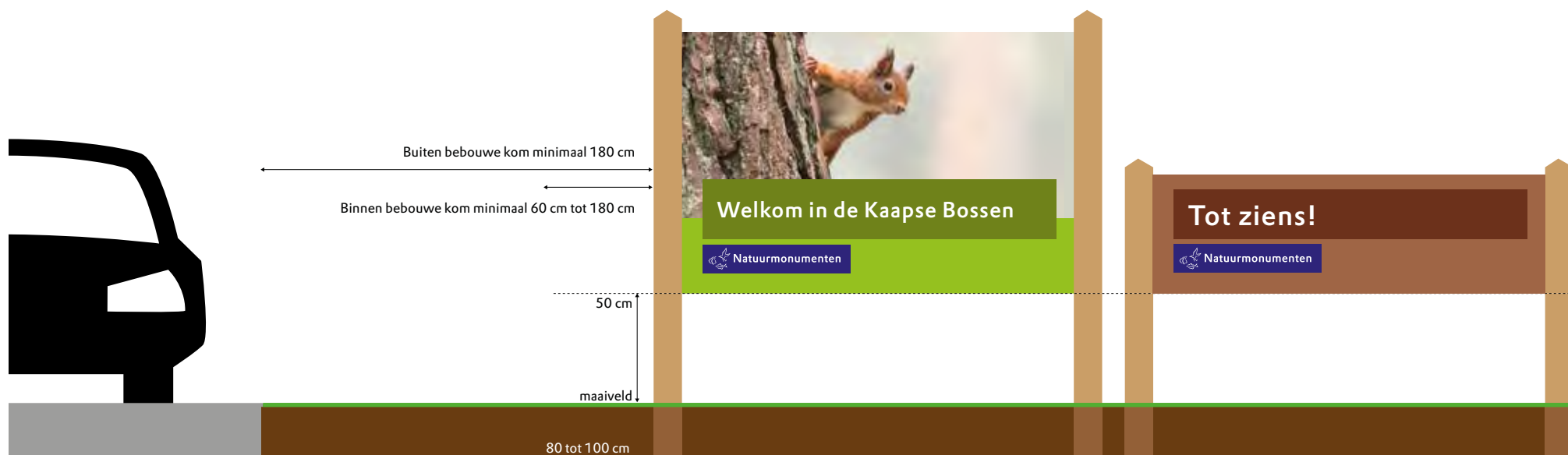
Entreebord groot 1-regelig 50 km 1800 x 1200 mm (standaard)
