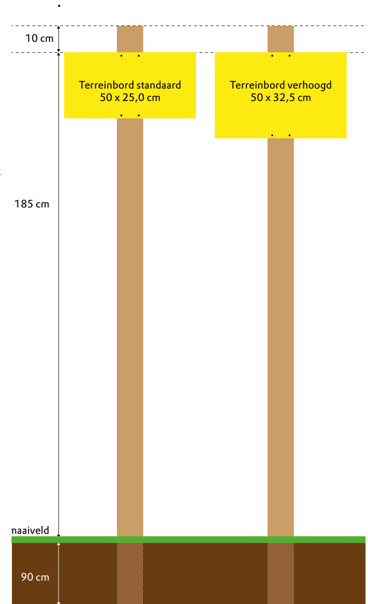
bovenaanzicht paal met terreinbord
