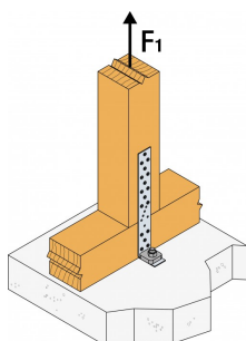
Fig. 1: Installasjon med én plate i bunnen, 45 mm
