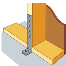
Fig. 1: Installasjon med én plate i bunnen, 45 mm
