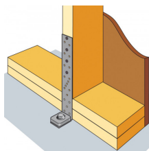
Fig. 2: Installasjon med to plater i bunnen, 45 mm
