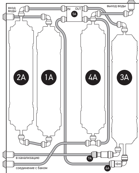
Рис. 2. Схема основного блока системы Expert Osmos M0510/M0520/M0530.
