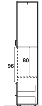
SEZIONE Section
