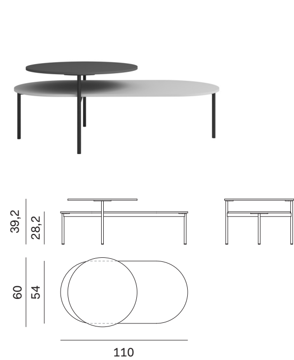
Tavolino L. 110 110cm-wide coffee table
