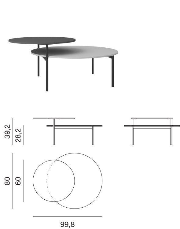
Tavolino L. 99,8 99,8cm-wide coffee table
