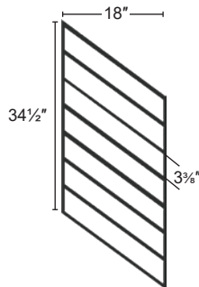
PR-O1836 22 1/2" Actual Rake Length
