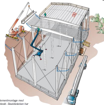
Takelementmontage med skyddsnet. Skyddsräcken har monterats på marken redan före lyft.
