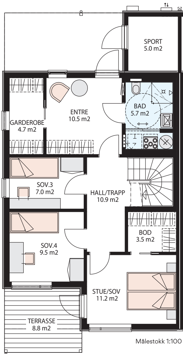
1. etasje
