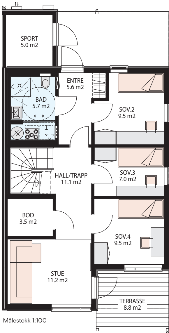
1. etasje
