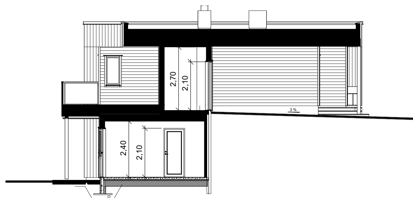
Snitt A-A
