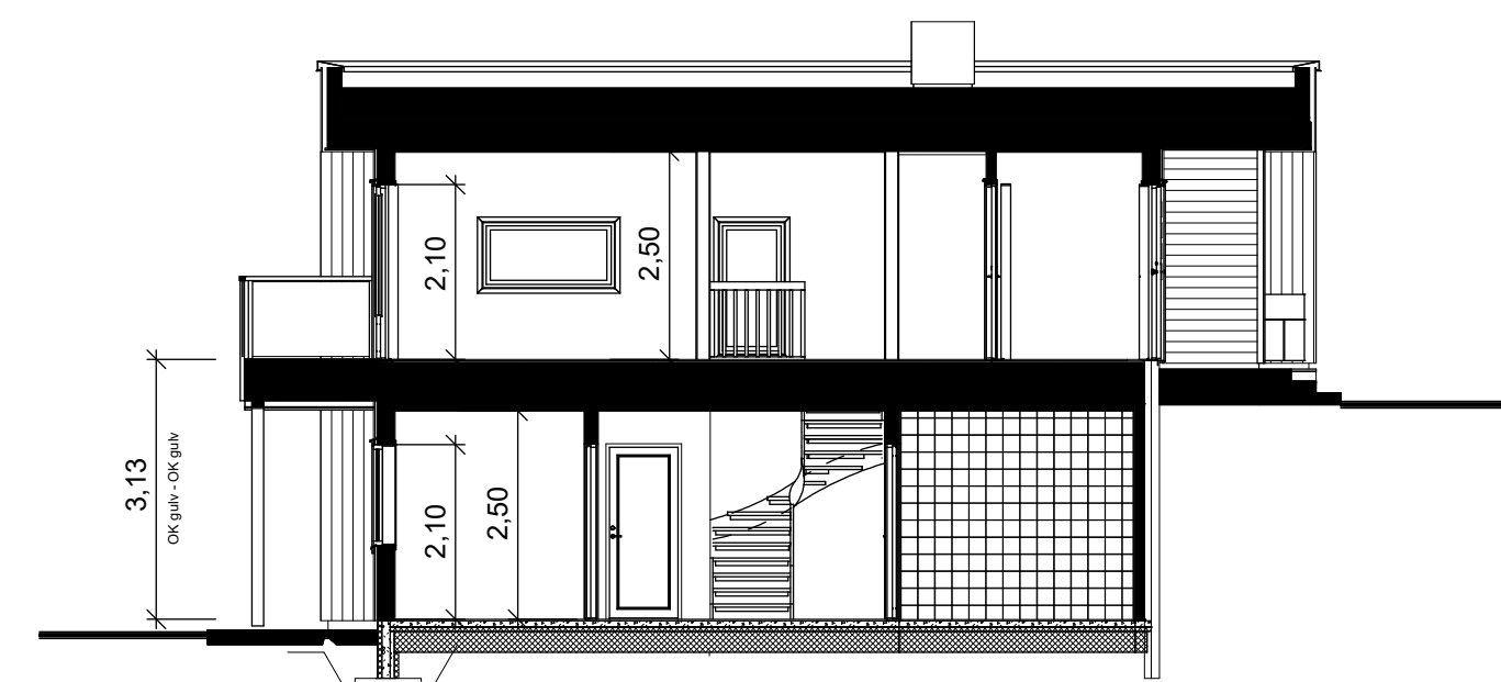
Snitt B-B
