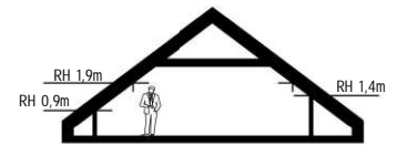
VINDSEKTION A2 SKALA 1 : 300
