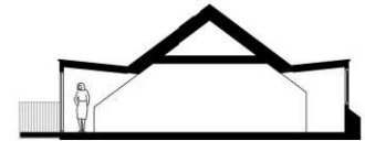
VINDSEKTION KUPA D2 SKALA 1 : 300
