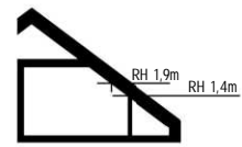
VINDSEKTION C2 SKALA 1 : 300
