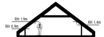
VINDSEKTION F1 SKALA 1 : 300
