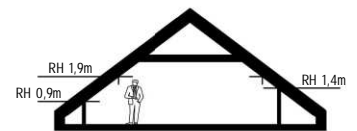
VINDSEKTION E1 SKALA 1 : 300
