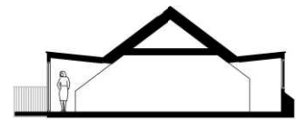
VINDSEKTION KUPA C1 SKALA 1 : 300
