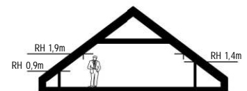
VINDSEKTION F2 SKALA 1 : 300
