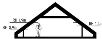
VINDSEKTION D1 SKALA 1 : 300
