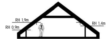
VINDSEKTION B2 SKALA 1 : 300
