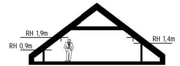
VINDSEKTION B1 SKALA 1 : 300
