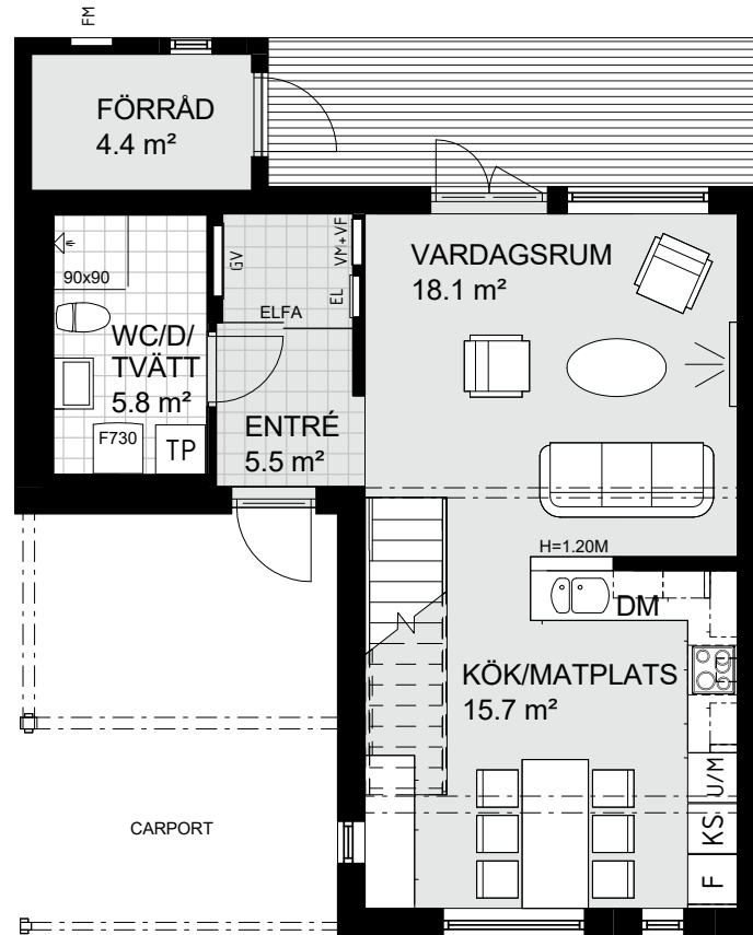
ENTRÉVÅNING
