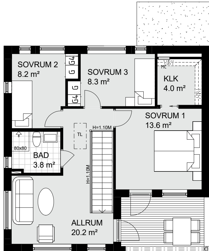
ÖVERVÅNING
