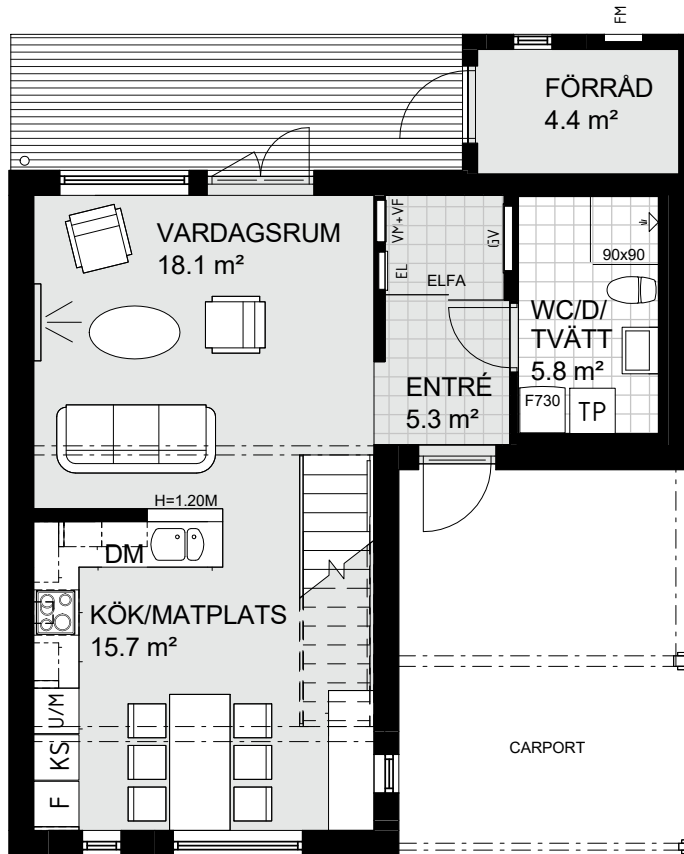
ENTRÉVÅNING
