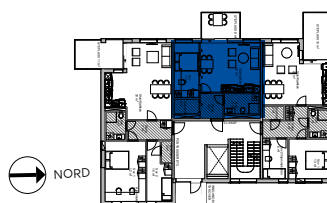
Etasjeplan
