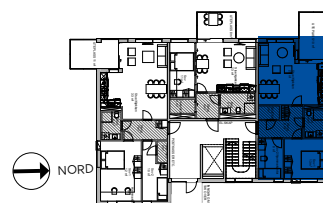
Etasjeplan
