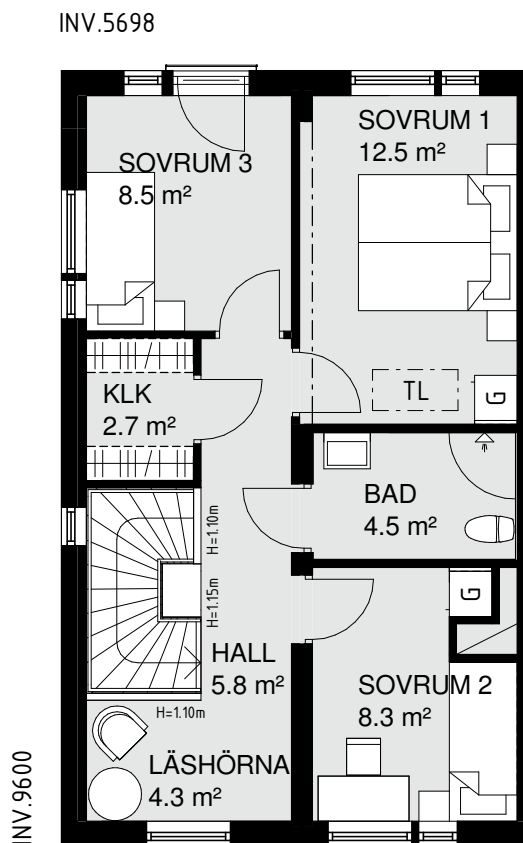
ÖVERVÅNING
