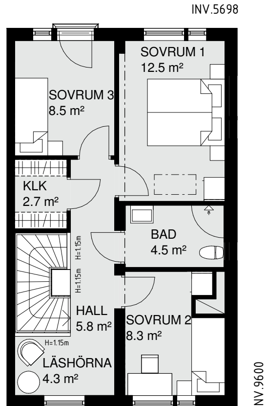
ÖVERVÅNING
