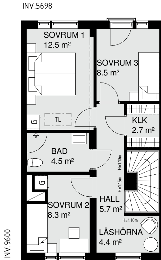
ÖVERVÅNING
