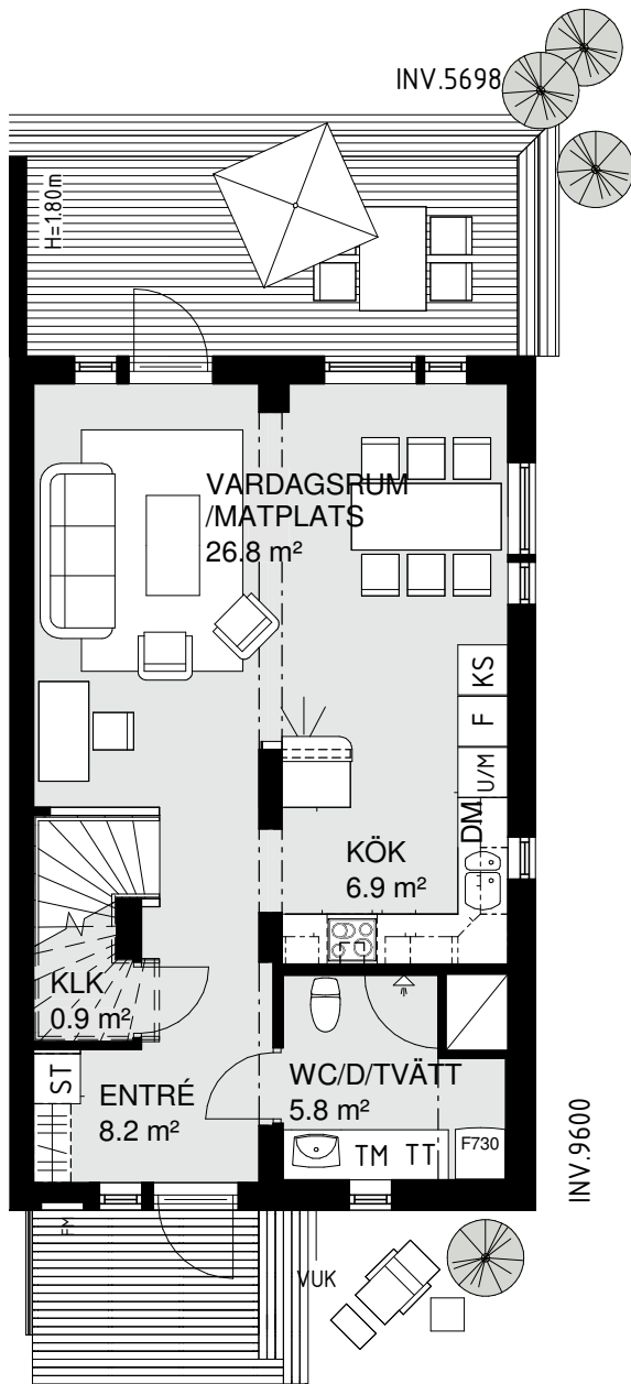
ENTRÉVÅNING
