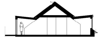
VINDSEKTION KUPA A1 SKALA 1 : 300
