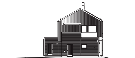
Fasade mot syd
