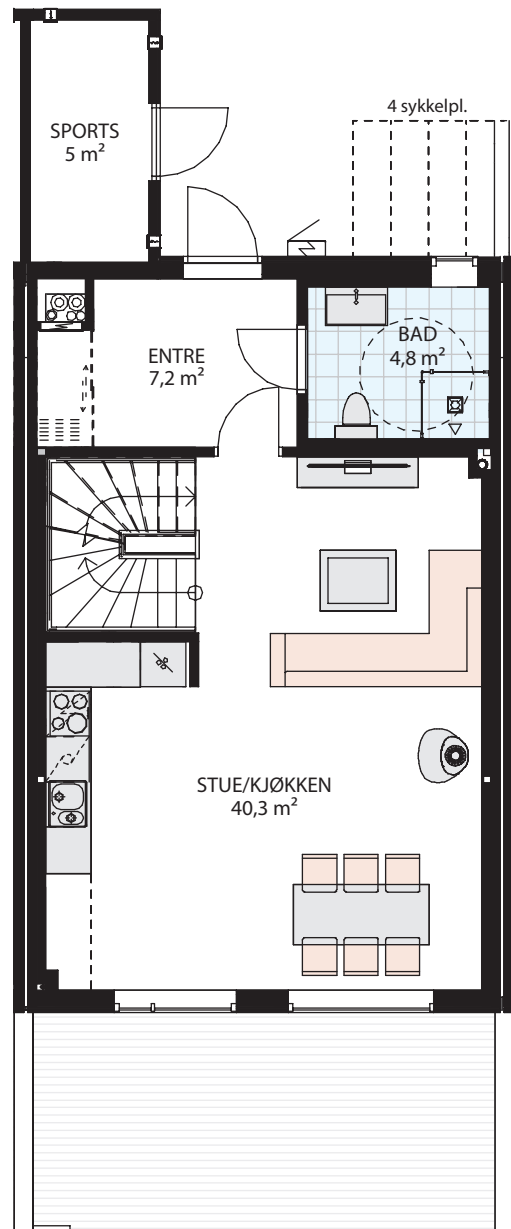
1. etasje
