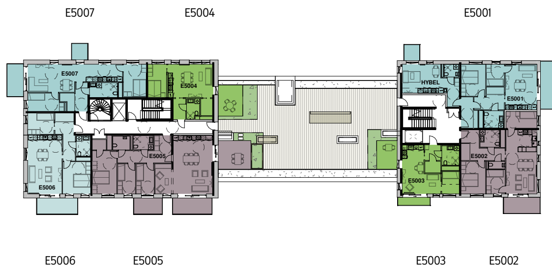
BYGG E, PLAN 5
