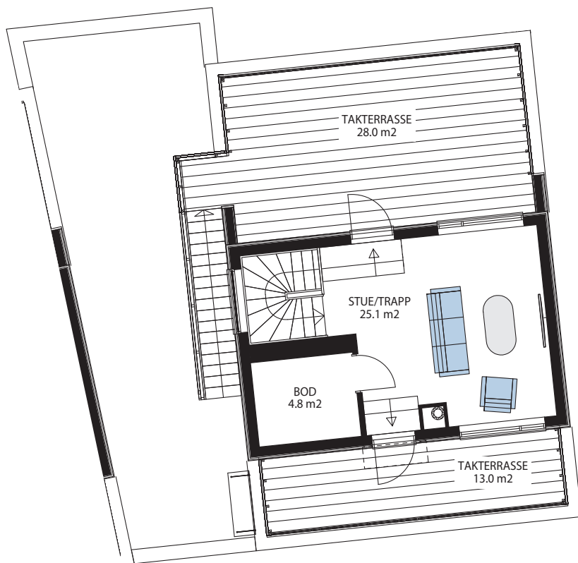
2. etasje
