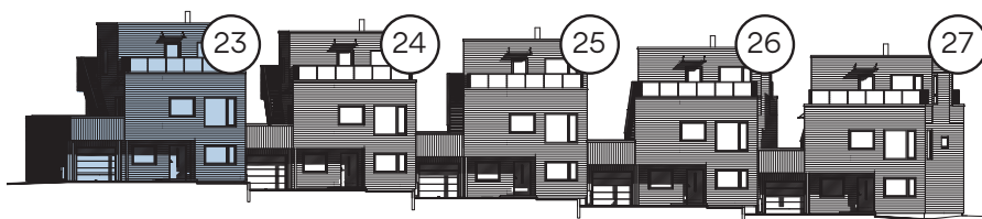
FASADE MOT NORD ØST
