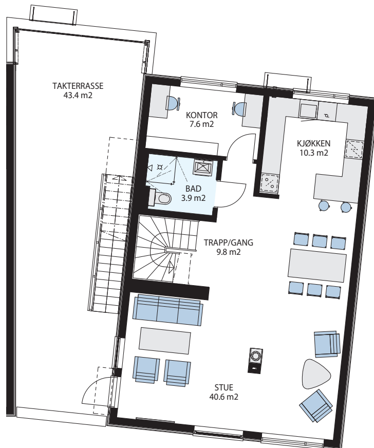
Målestokk 1:125
