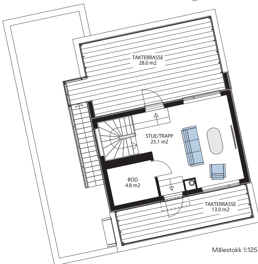
2. etasje
