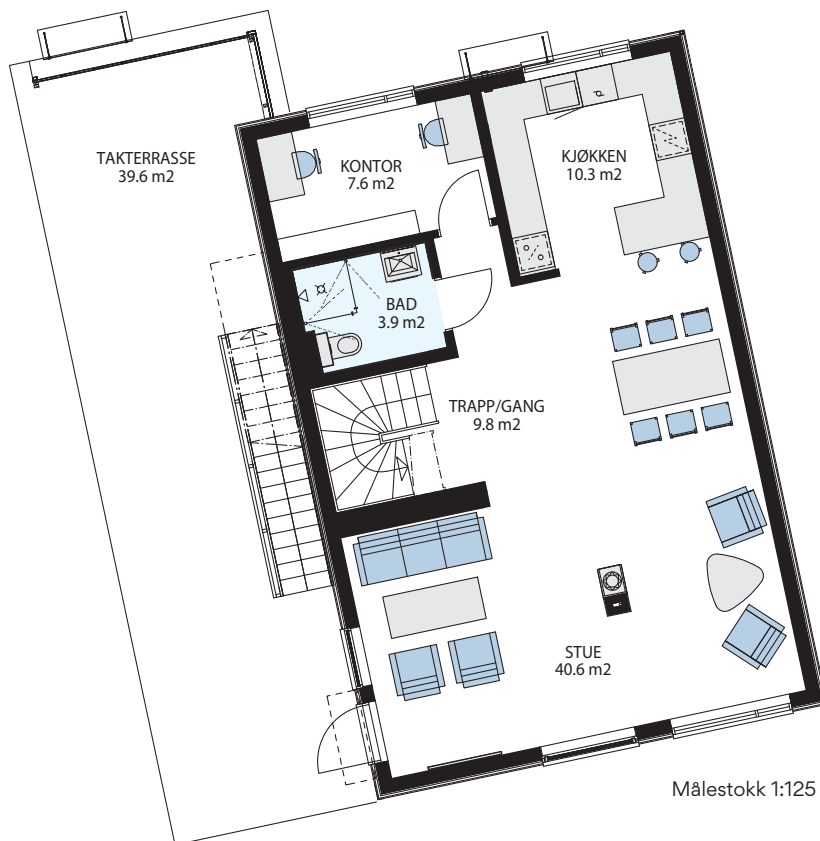
1. etasje
