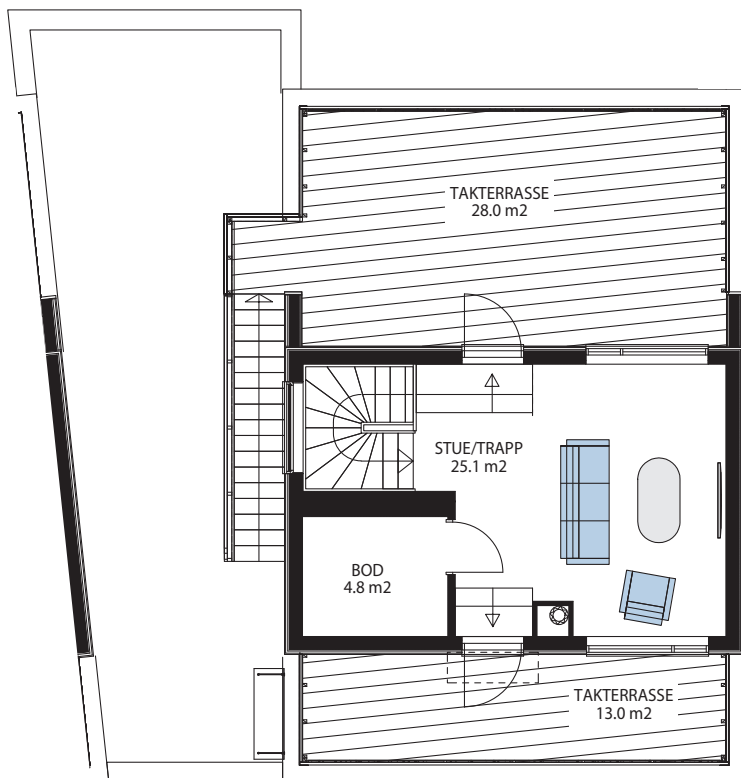
2. etasje
