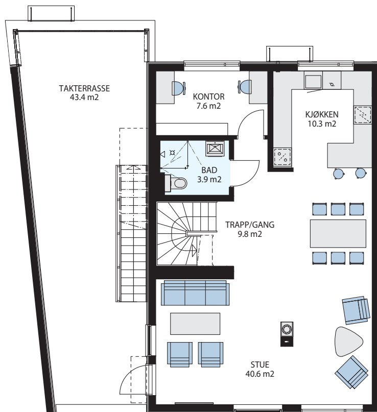
1. etasje
