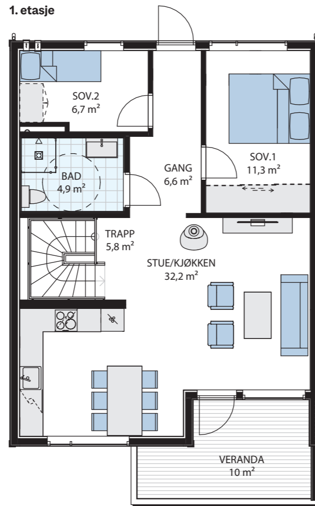
Målestokk 1:100
