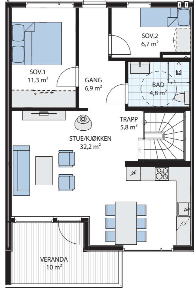
Målestokk 1:100
