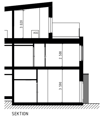
SEKTION
