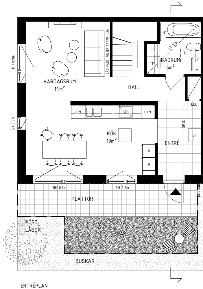
ENTRÉPLAN
