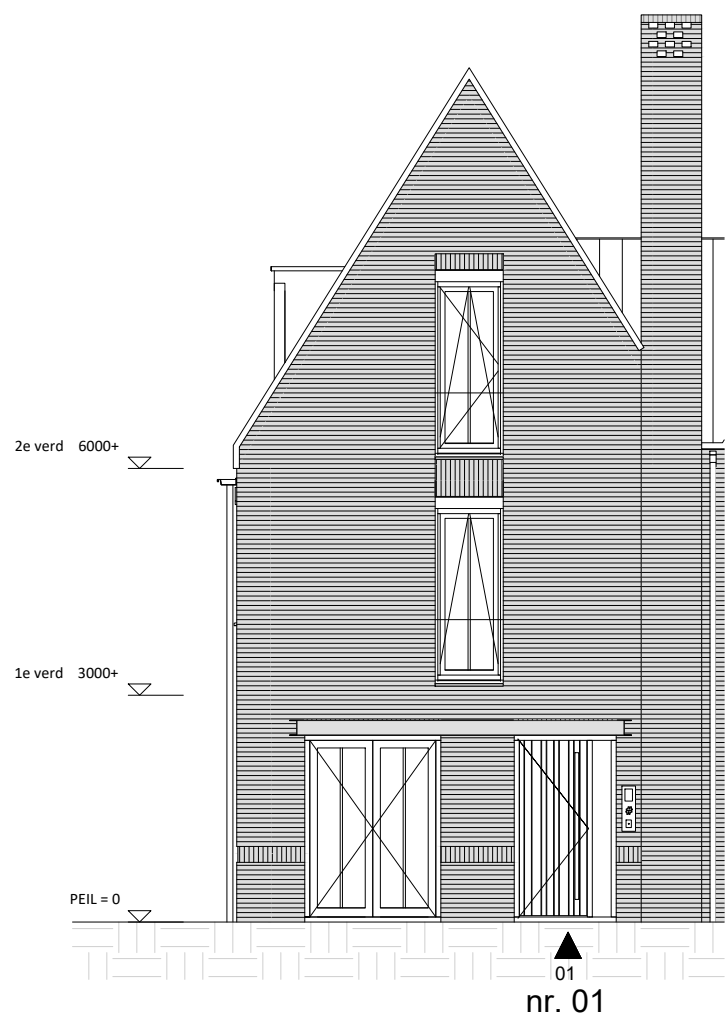
Voorgevel (oostgevel) 1:100
