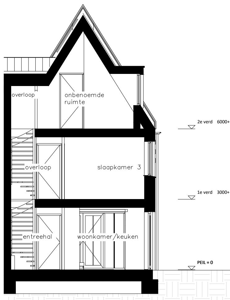
Doorsnede 1:100
