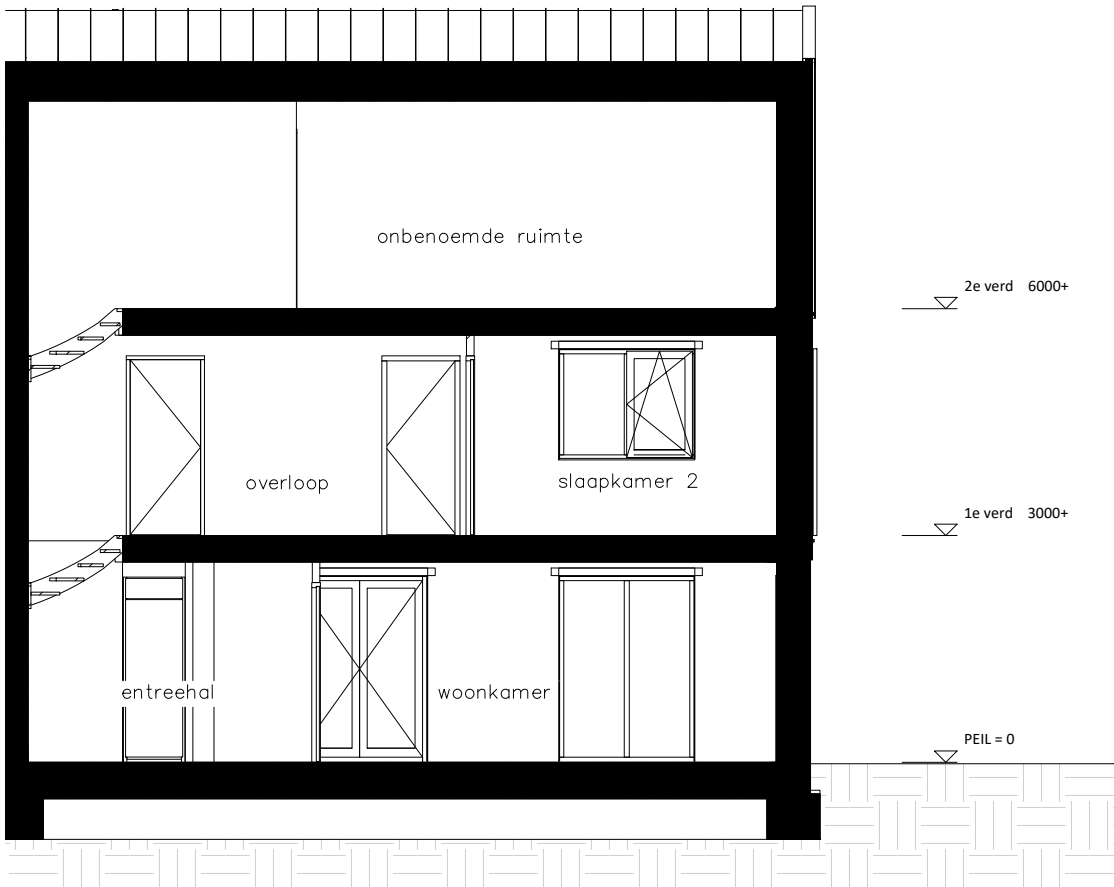
Doorsnede 1:100
