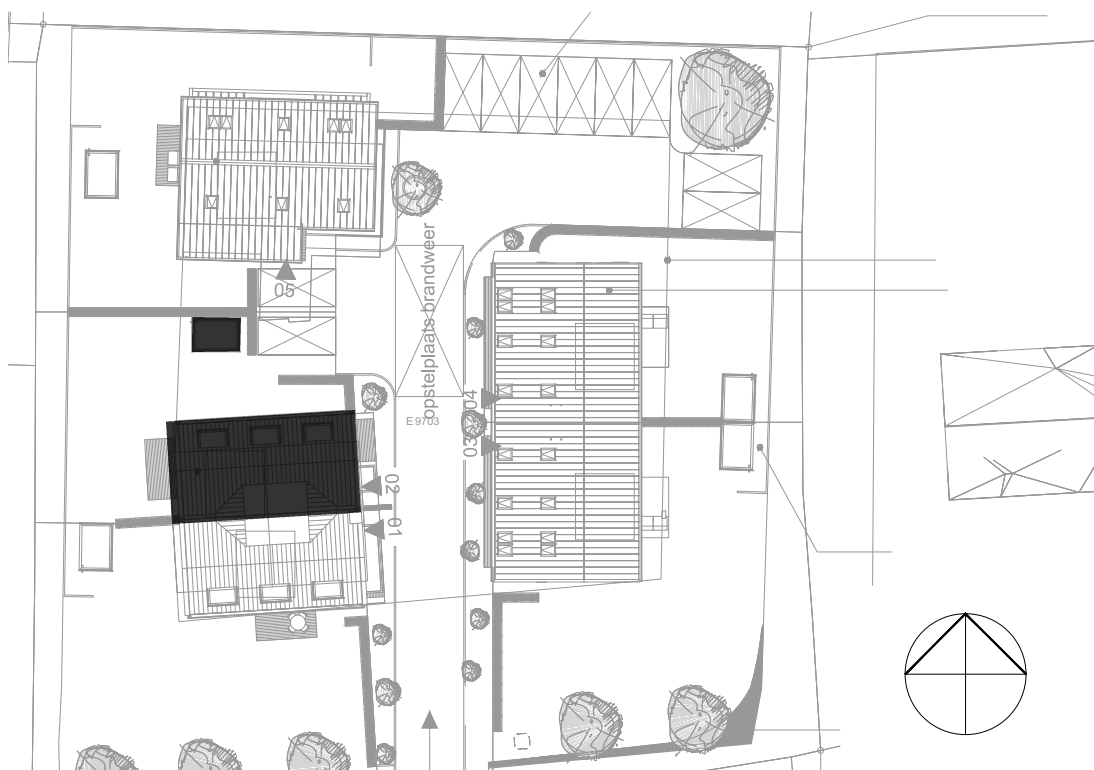
Situatie 1:500
