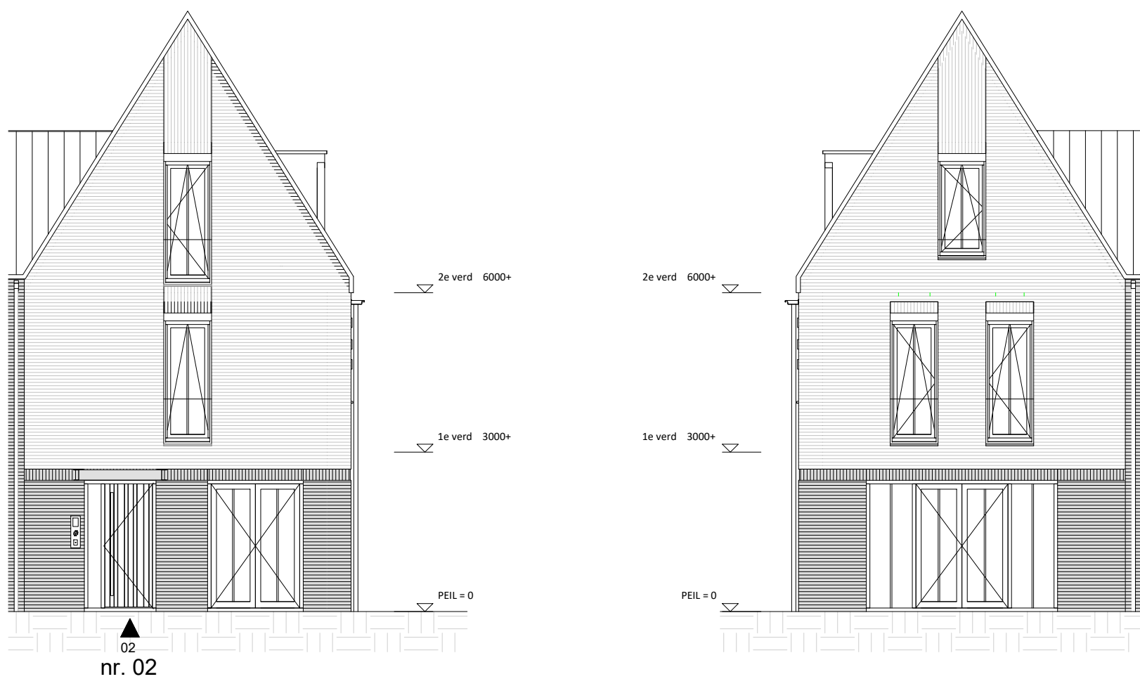
Voorgevel (oostgevel) 1:100
