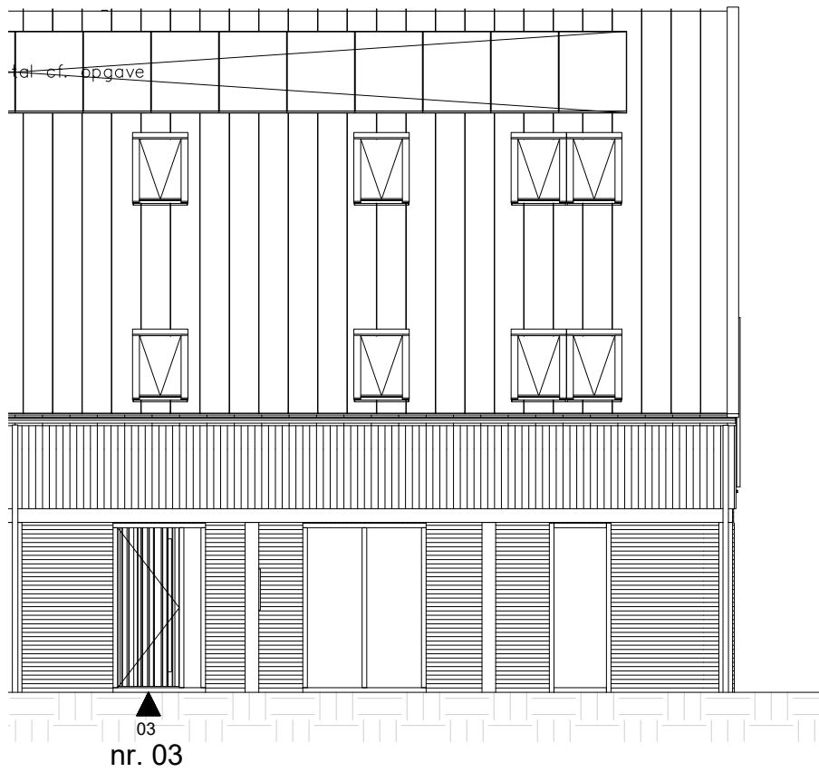
Voorgevel (westgevel) 1:100
