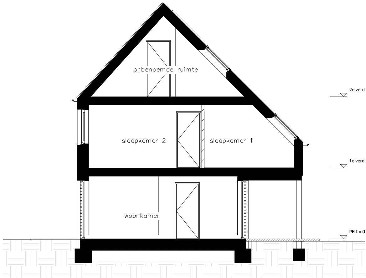
Doorsnede 1:100
