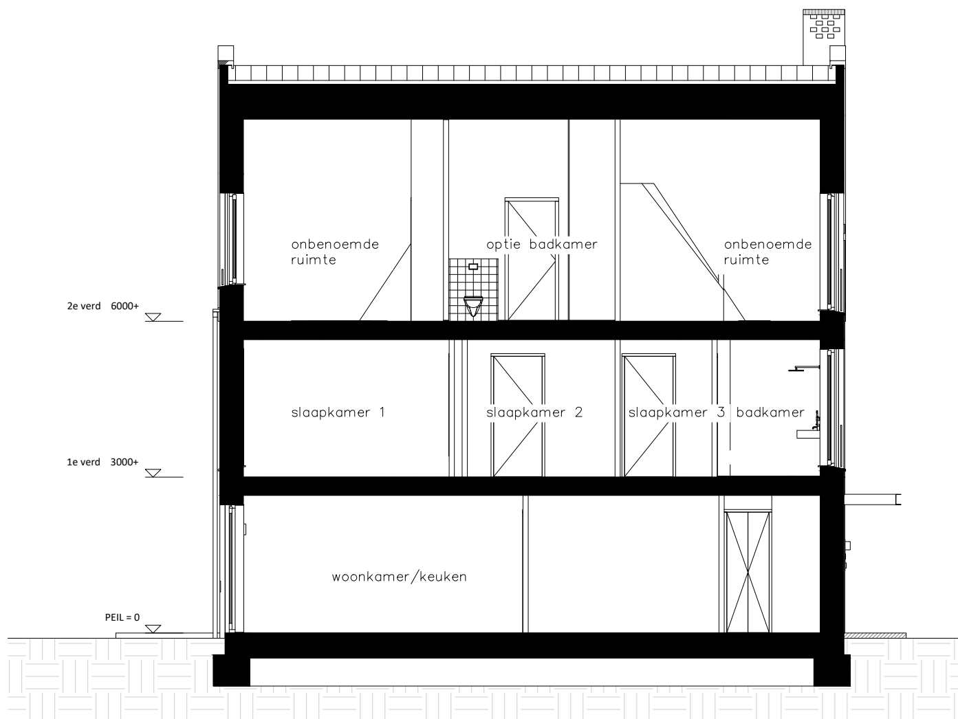
Doorsnede 1:100
