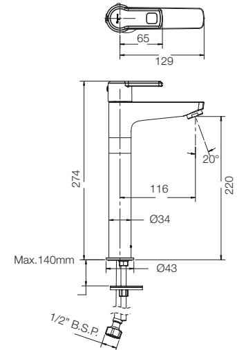
TALL PILLAR TAP G3942A1
