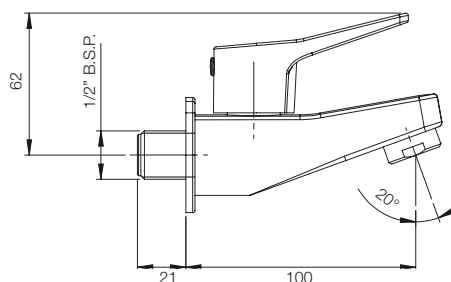
BIB COCK G5704A1
