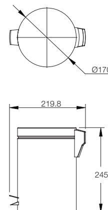
DUSTBIN 3L T6601A1
