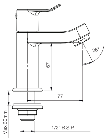
PILLAR TAP G2722A1
