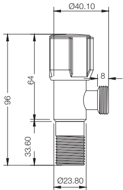
CASA (SS) T9886A1
