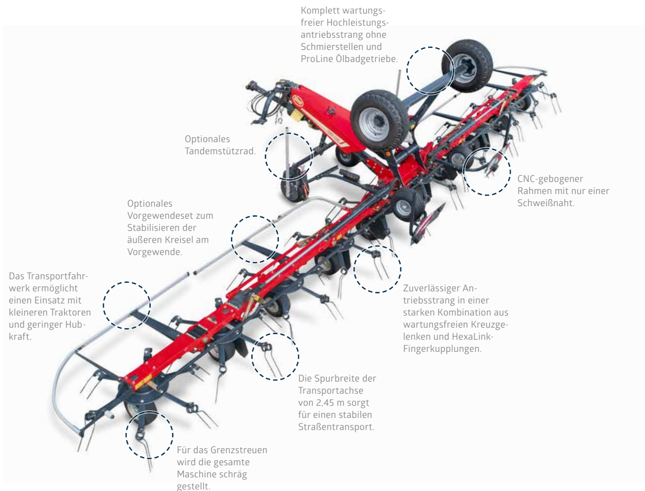
Optional ist ein Tandemstützrad an der Deichsel verfügbar.
