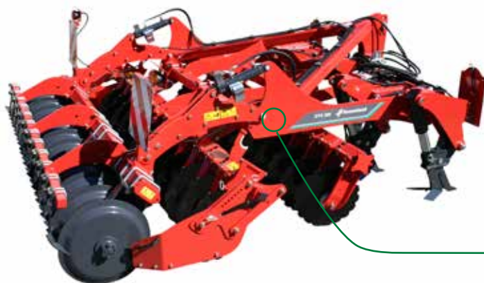
DTX 3.00 m; dent Pro-Lift profondeur de travail jusqu'à 40 cm; rangées de disques profondeur de travail de 2 à 10 cm.
