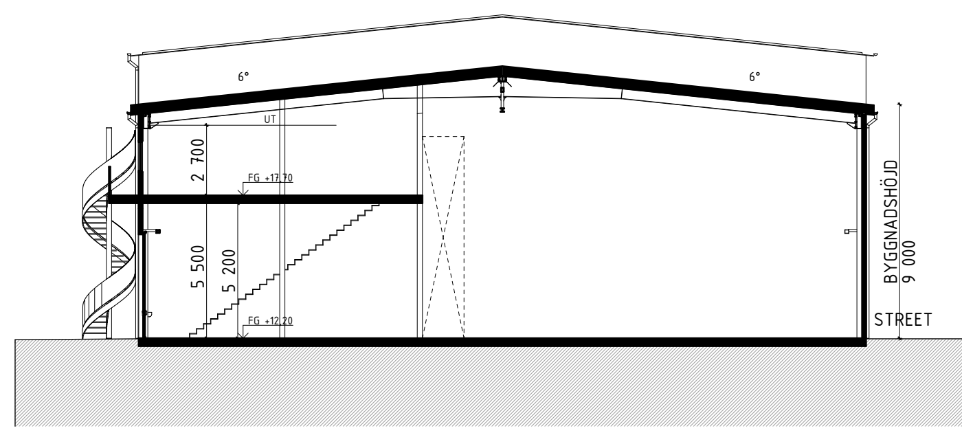
SEKTION 1:200
