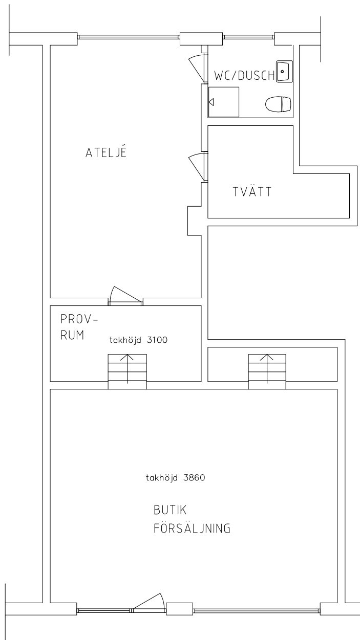
PLAN - KOBARNAS VÄG 4 - KLÄDBUTIK/ATELJÉ
